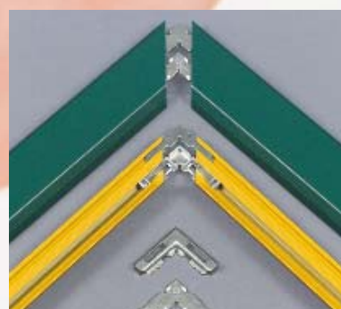
Az alumíniumkeret rendkívül stabil, erről a toknál és a szárnyánál is sarkonként két-két pánt gondoskodik. Ezek a pántok a sarkokat oldhatatlanul kötik össze.
