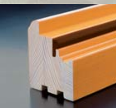
A lazúrréteget még az üvegezés és a vasalatok szerelése előtt felvisszük, így az egész felület védett.
